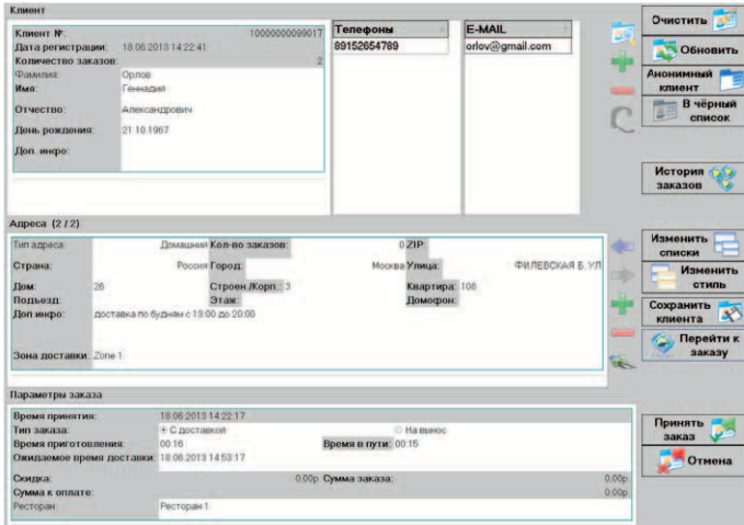
Прием заказов на доставку в модуле Оператор Delivery.
